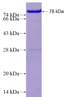
Recombinant Human SPARCL1 SDS-PAGE
