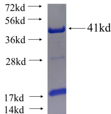
Recombinant human KIAA1217 SDS-PAGE
