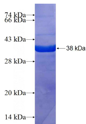
Recombinant Human SDCBP2 SDS-PAGE
