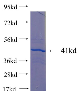
Recombinant human C6orf125 SDS-PAGE
