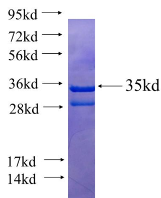
Recombinant human MIP SDS-PAGE
