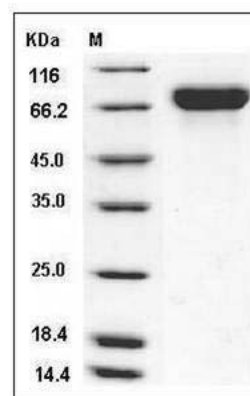
Influenza A H1N1 (A/Texas/05/2009) Hemagglutinin / HA Protein (His Tag) SDS-PAGE
