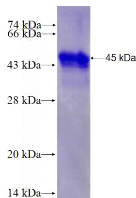
Recombinant Human IL-11RA SDS-PAGE
