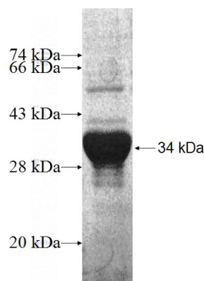
Recombinant Human NTAN1 SDS-PAGE
