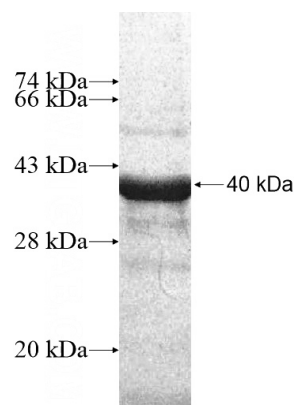
Recombinant Human KIF19 SDS-PAGE
