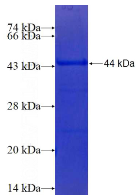
Recombinant Human TRPS1 SDS-PAGE
