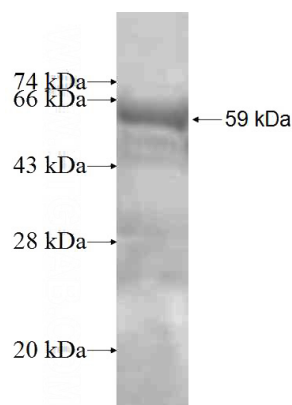
Recombinant Human NMRAL1 SDS-PAGE
