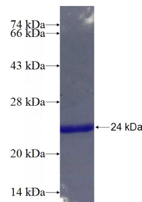
Recombinant Human SH3BP5L SDS-PAGE
