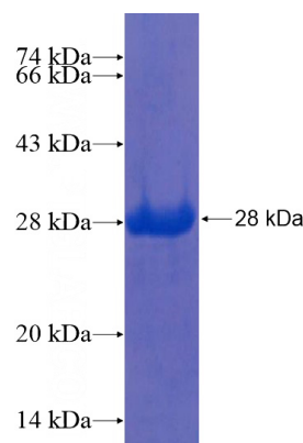
Recombinant Human PLAA SDS-PAGE
