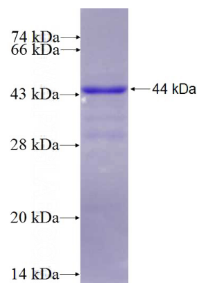
Recombinant Human RCBTB2 SDS-PAGE
