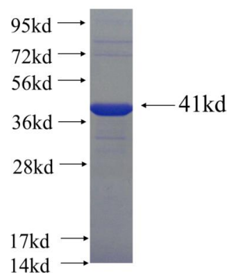
Recombinant Arabidopsis thaliana EVR SDS-PAGE
