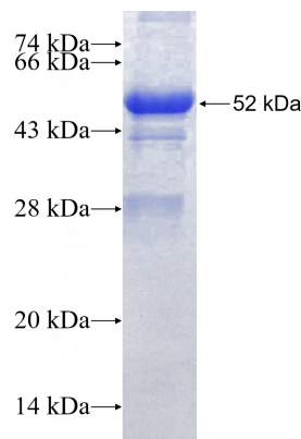
Recombinant Human P53 SDS-PAGE
