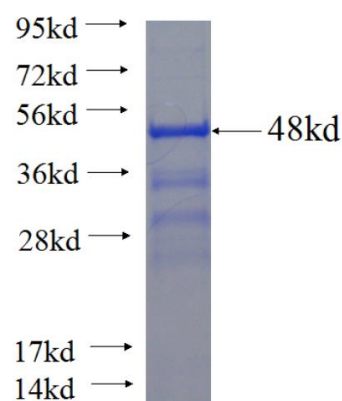
Recombinant human TRPV1 SDS-PAGE
