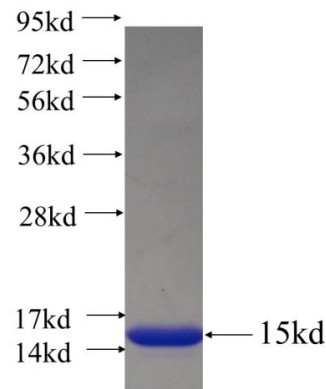
Recombinant human C14orf159 SDS-PAGE
