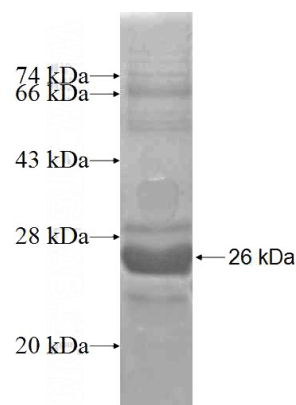
Recombinant Human NIPBL SDS-PAGE
