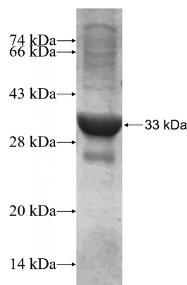
Recombinant Human REDD1 SDS-PAGE
