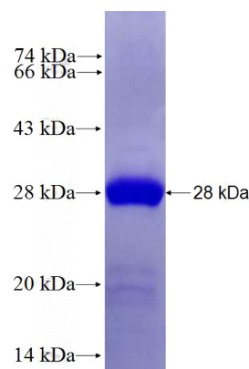
Recombinant Human TRAPPC4 SDS-PAGE
