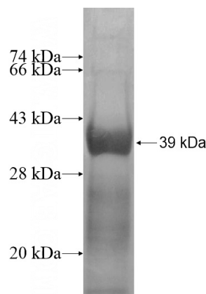
Recombinant Human OPHN1 SDS-PAGE
