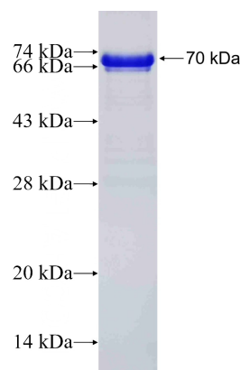
Recombinant human NRF2, NFE2L2 SDS-PAGE
