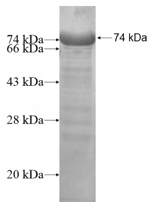
Recombinant Human KIAA1430 SDS-PAGE
