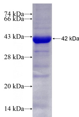
Recombinant Human NXF1 SDS-PAGE
