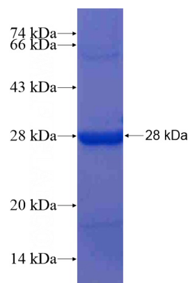
Recombinant Human JTV1 SDS-PAGE
