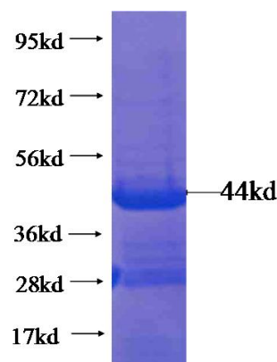
Recombinant human C9orf41 SDS-PAGE
