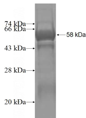
Recombinant Human E2F6 SDS-PAGE
