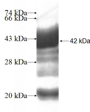
Recombinant Human UBXN6 SDS-PAGE
