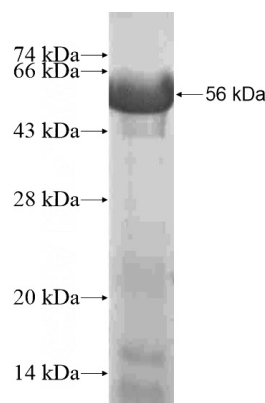
Recombinant Human TCHHL1 SDS-PAGE
