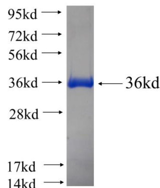
Recombinant human HMG20B SDS-PAGE
