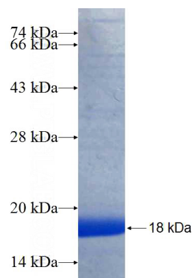
Recombinant Human VHL SDS-PAGE
