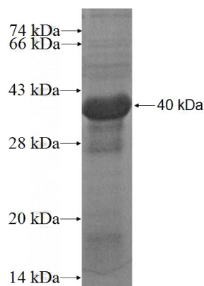
Recombinant Human C10orf119 SDS-PAGE
