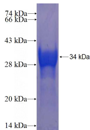
Recombinant Human PDS5B SDS-PAGE
