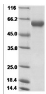
H10N7 HA Protein 14768
