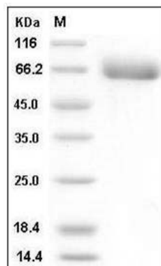
Human EphA4 Protein (His Tag) SDS-PAGE
