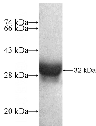
Recombinant Human DISP1 SDS-PAGE
