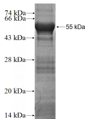
Recombinant Human MAF1 SDS-PAGE
