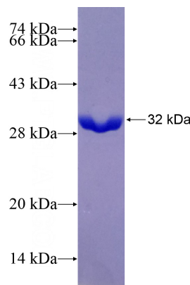
Recombinant Human filamin-c SDS-PAGE
