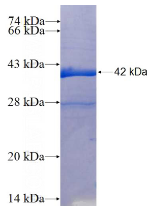
Recombinant Human TAF5 SDS-PAGE
