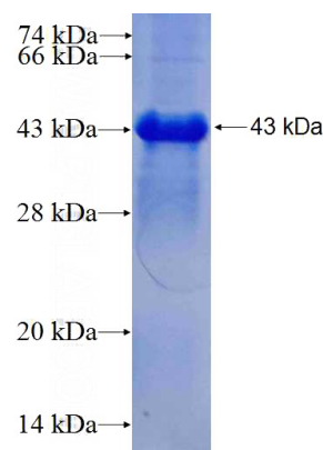
Recombinant Human ANKRD17 SDS-PAGE
