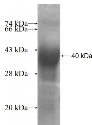
Recombinant Human LLGL2 SDS-PAGE
