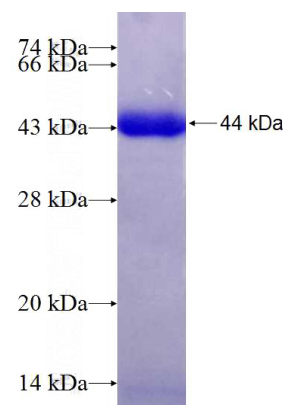
Recombinant Human CHAT SDS-PAGE
