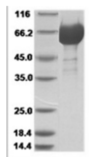
H1N1 HA Protein 14129
