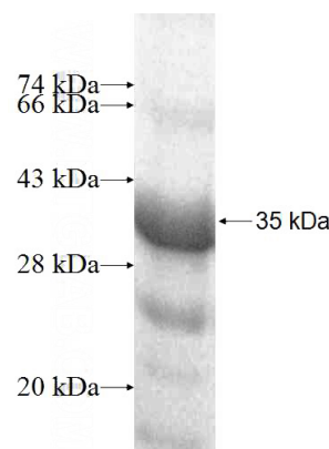
Recombinant Human MESP1 SDS-PAGE
