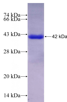
Recombinant Human CKAP4 SDS-PAGE
