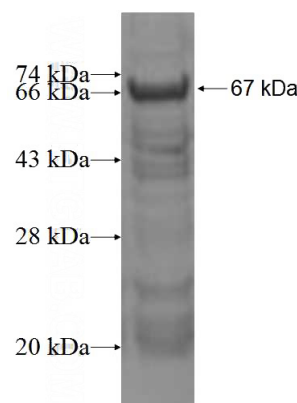
Recombinant Human CNNM4 SDS-PAGE
