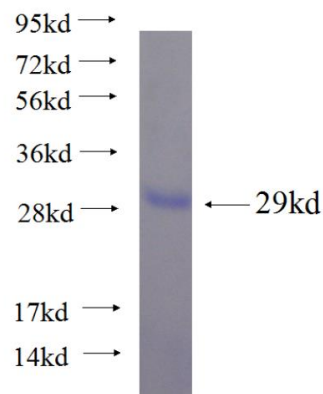
Recombinant human C10orf107 SDS-PAGE
