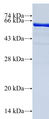
Recombinant Human PAOX SDS-PAGE
