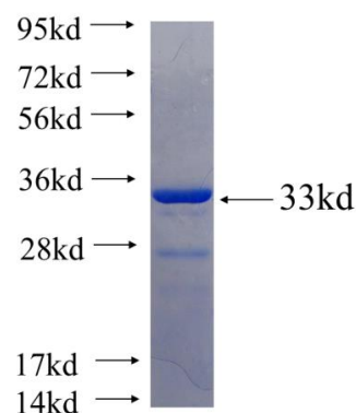
Recombinant human C20orf11 SDS-PAGE
